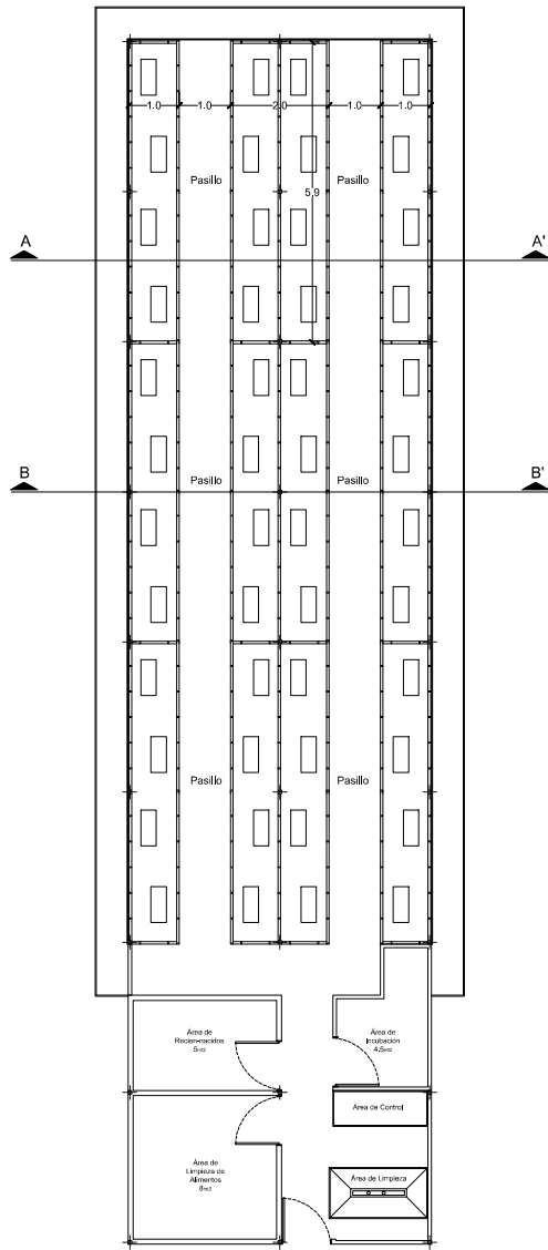
Planta Distribución Módulos de 3x3 propuestos Esc: 1/100
