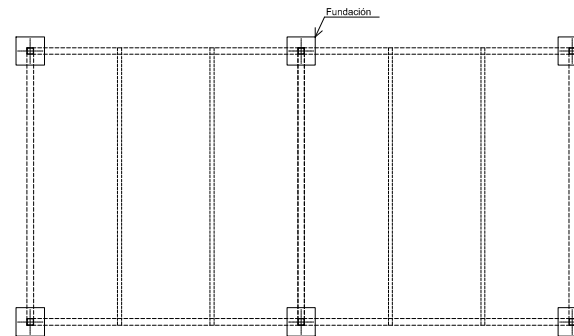
Planta Diseño Módulo Estructural Esc: 1/50
