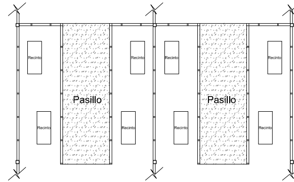
Planta - Módulo 3x3 Áreas de engorde Esc: 1/50
