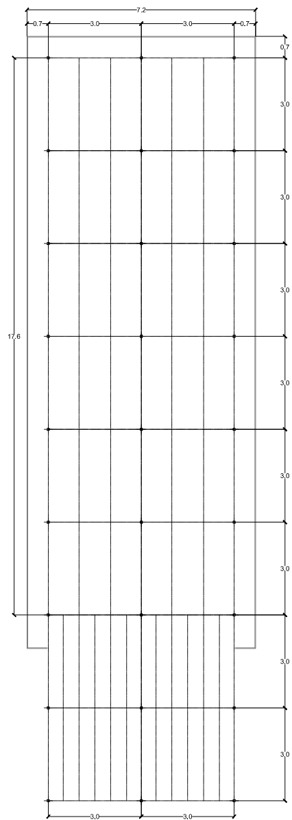
Planta Estructura Esc: 1/100
