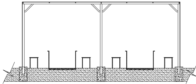
Sección B-B' Áreas de engorde
