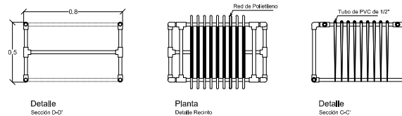
Detalles Recintos Esc: 1/25
