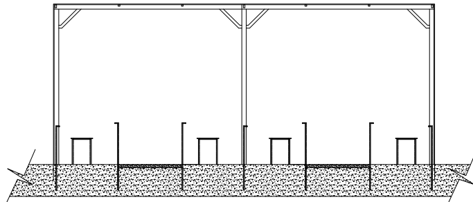
Sección A-A' Áreas de engorde
